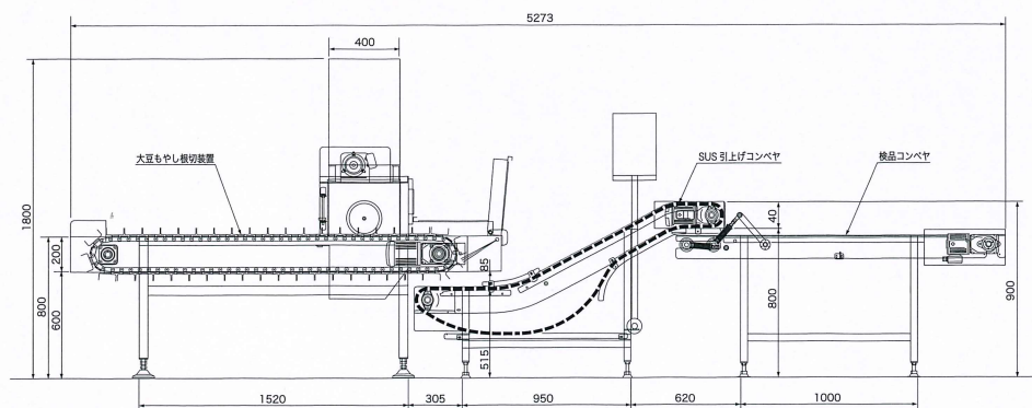
■コンベヤ搬送式 大豆もやし根切機の設置寸法例 ★図は根切り検品ライン例
