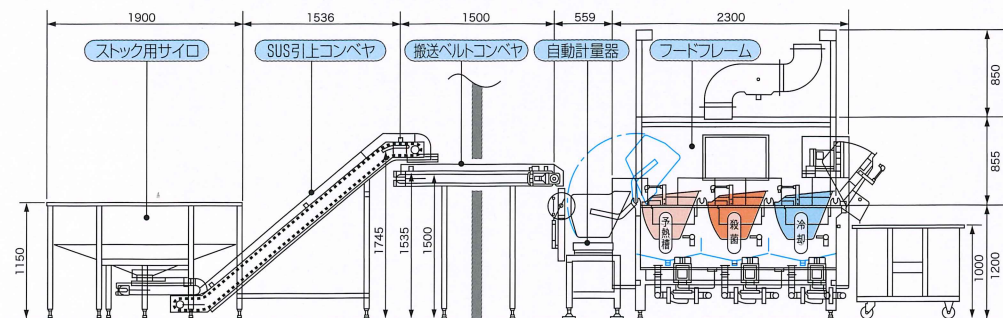
■バスケットシリンダー反転式 種子加熱殺菌装置の設置寸法例
