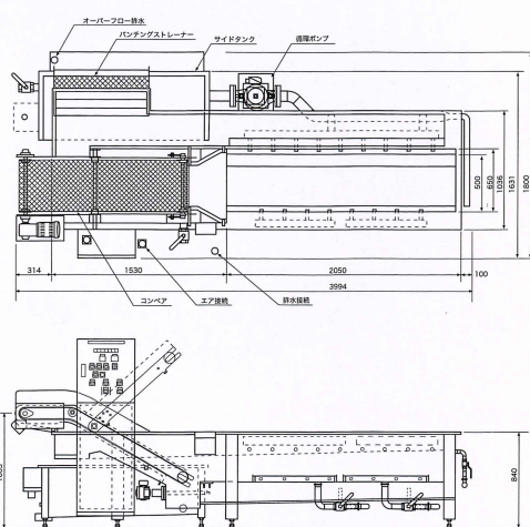
■機械寸法図と各名称 (SPW-6)
